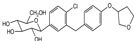
Fig. 1. Empagliflozin
